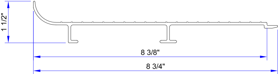
1 1/2 x 8 IL-RISER ( ALCOA # 68194 )
