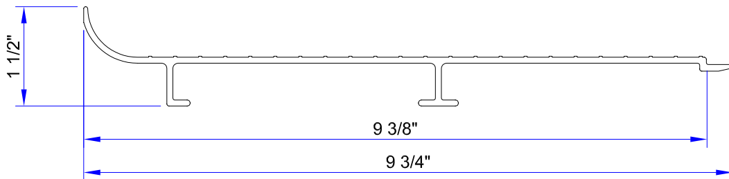
1 1/2 x 9 IL-RISER ( ALCOA # 68395 )
