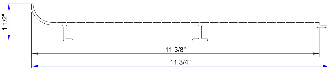
1 1/2 x 11 IL-RISER ( ALCOA # 68106 )
