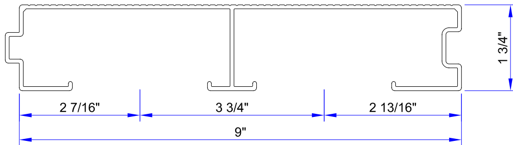
2 x 9 IL-DECK ( ALCOA # 69964 )
