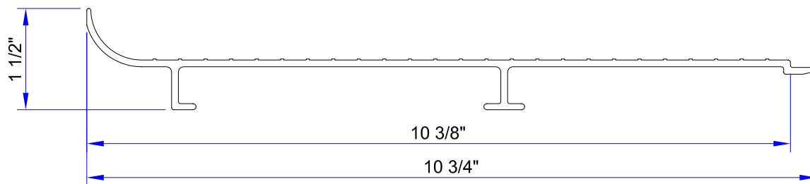
1 1/2 x 10 IL-RISER ( ALCOA # 68105 )
