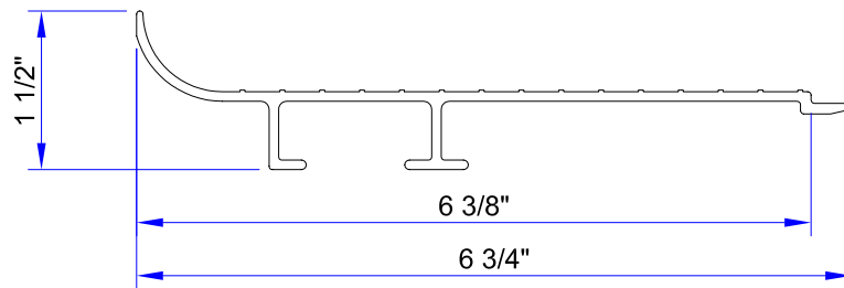
1 1/2 x 6 IL-RISER ( ALCOA # 68195 )
