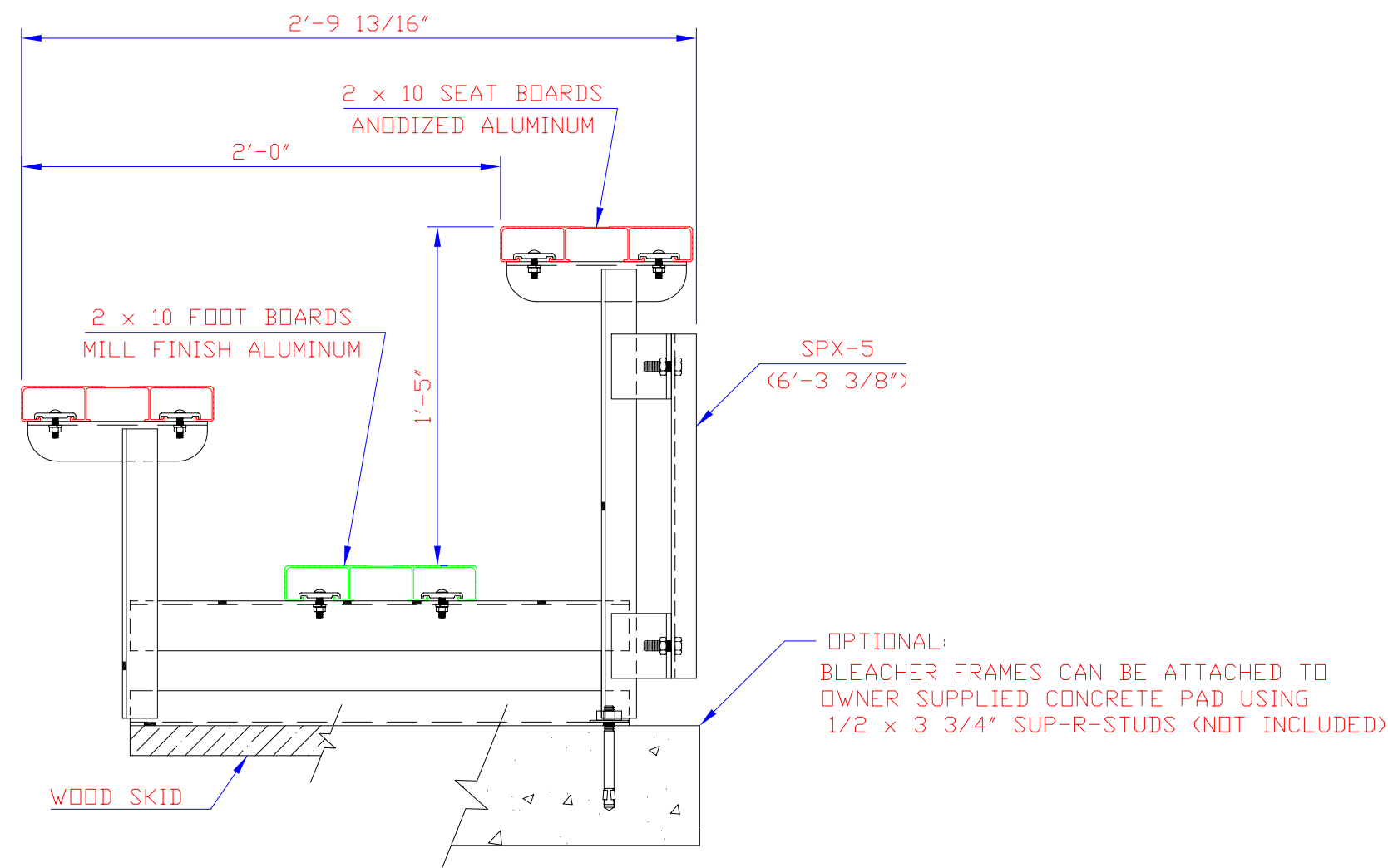
END ELEVATION
