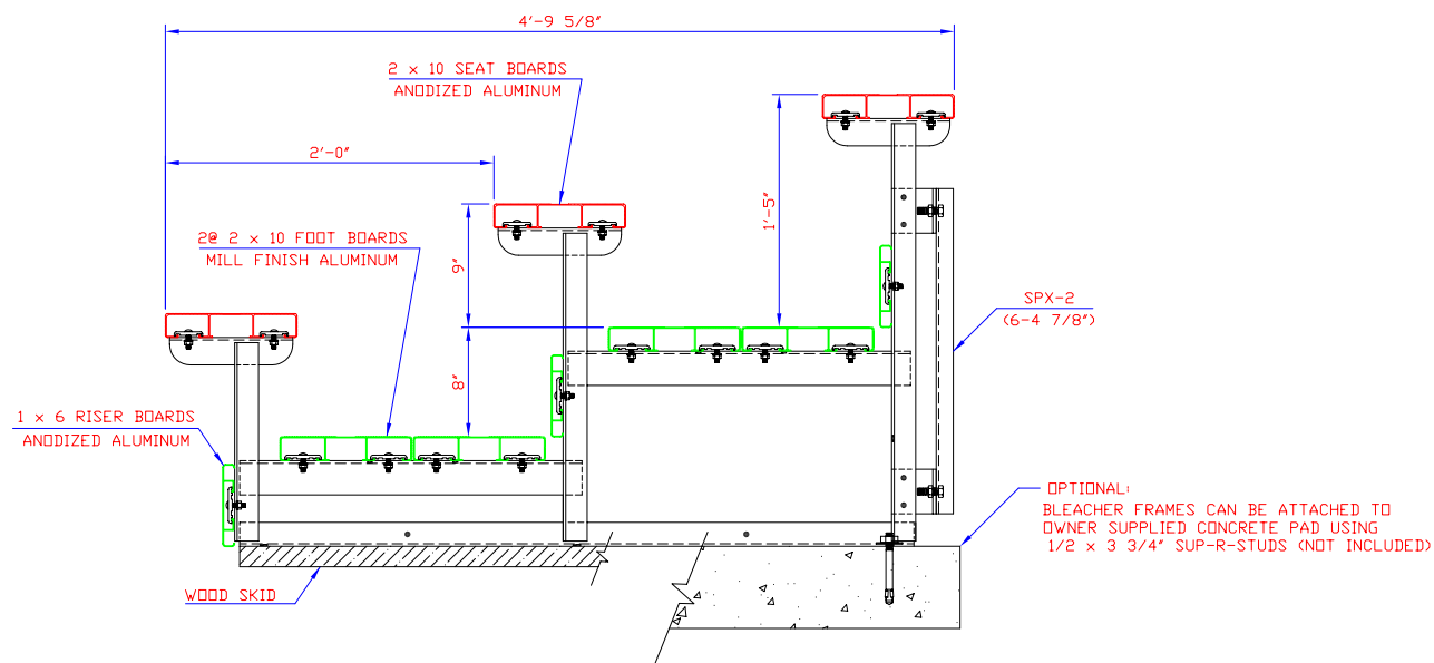
END ELEVATION
