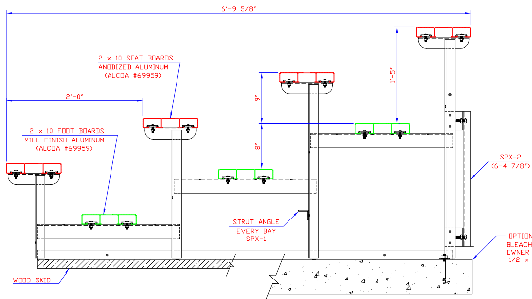
END ELEVATION
